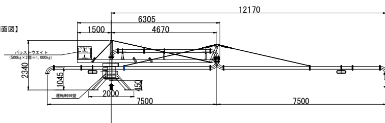
【正面図】
