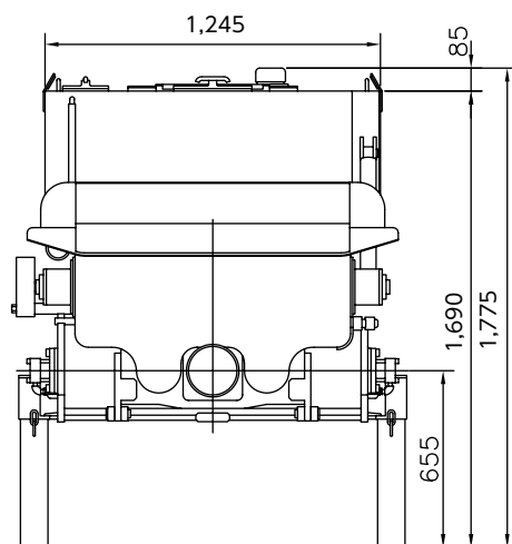
MKW-35SM外観図
