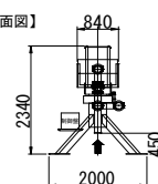
【正面図】
