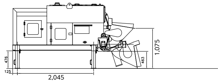
外寸図
