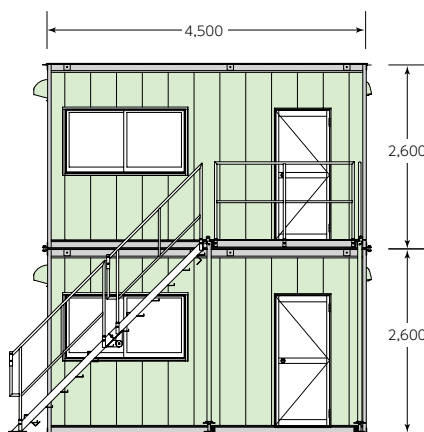
▲RS-30 2階建てタイプ
