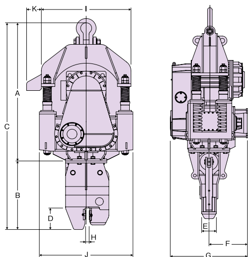
◎寸法図(ZERO-MR)
