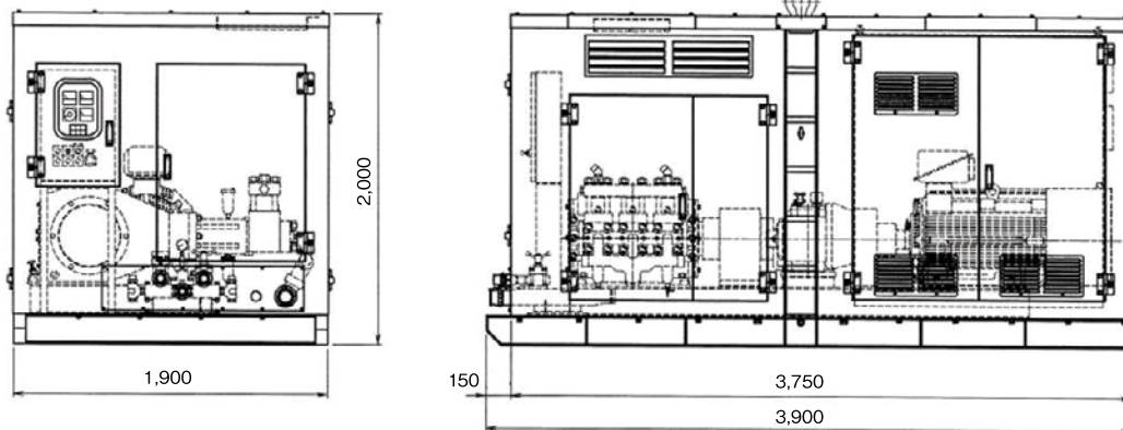
◎寸法図
