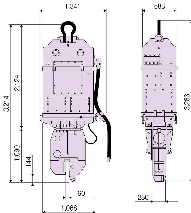
◎寸法図
