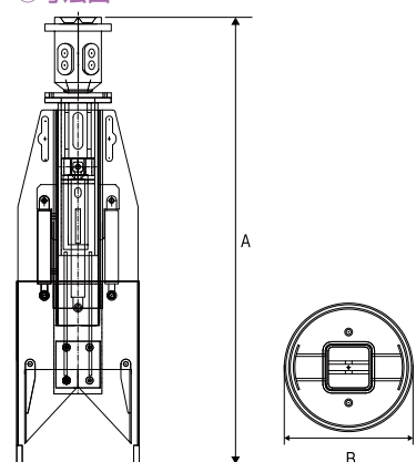
◎寸法図
